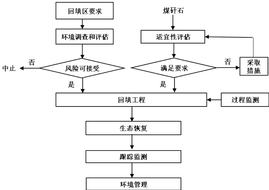
图 A.1 煤矸石生态回填流程图
